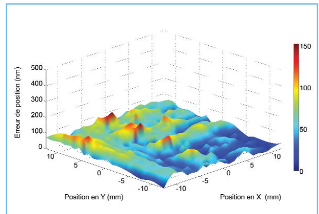
ANT95-XY PLUS Précision en 2D
