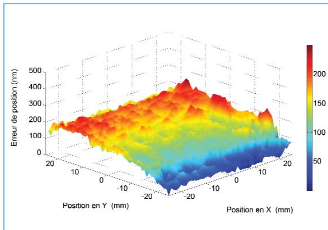
ANT130-XY PLUS Précision en 2D
