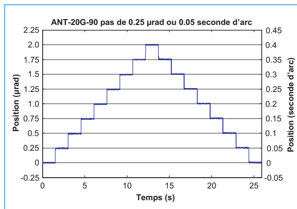
ANT-20G-90 pas de 0.05 seconde d'arc
