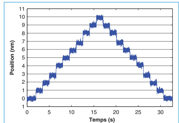
ANT130-060-L-PLUS Pas de 1 nm
