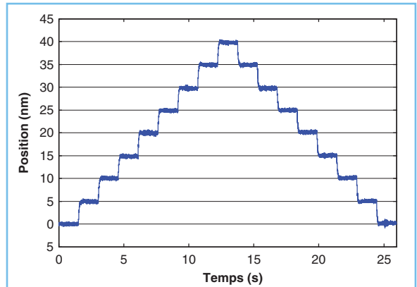
ANT95-50-L-Z-PLUS Pas de 5 nm
