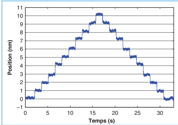
ANT95-50-L-PLUS pas de 1 nm
