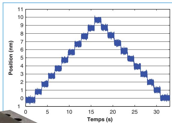
ANT95-3-V Pas de 1 nm
