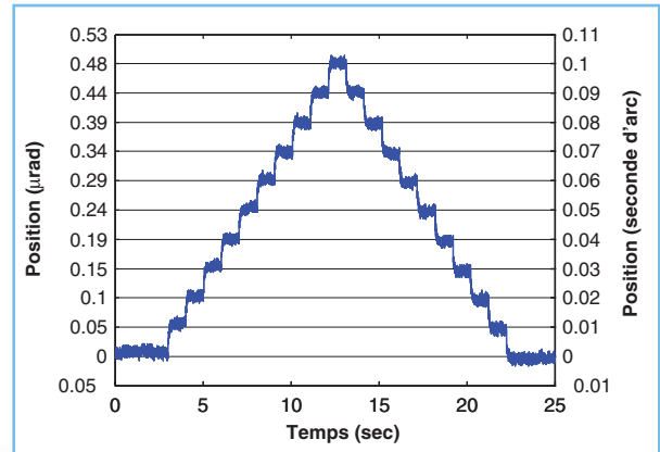
ANT95-R pas de 0.01 seconde d'arc
